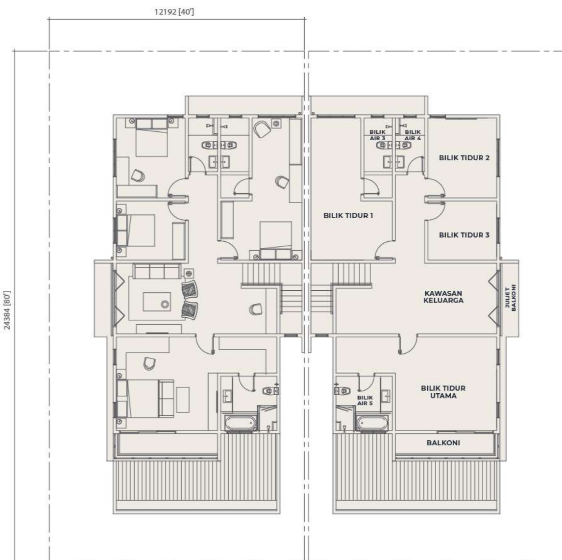
TINGKAT ATAS
