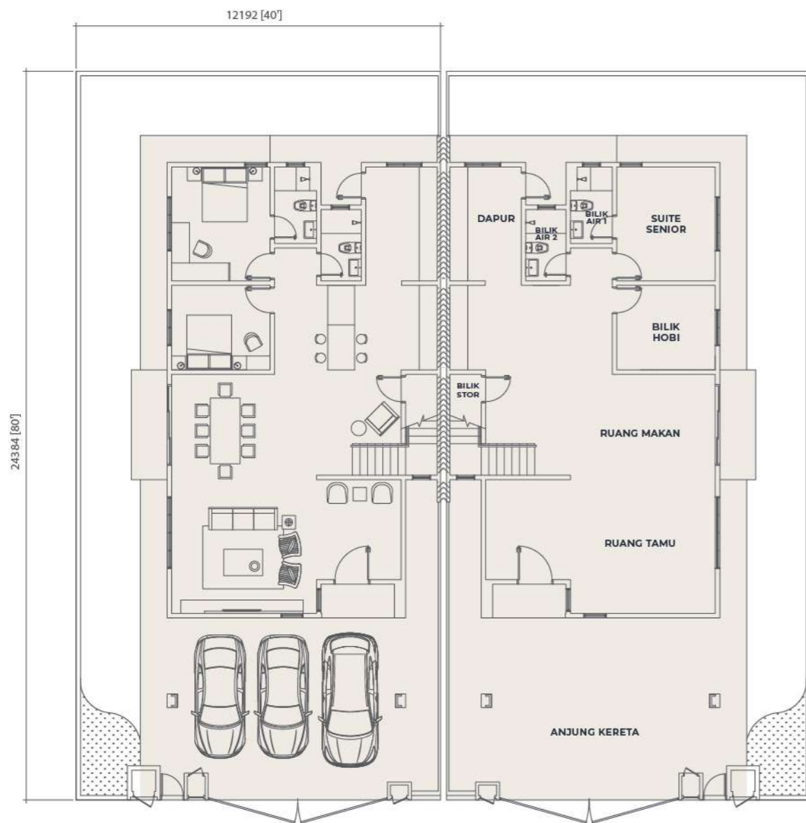
TINGKAT BAWAH
